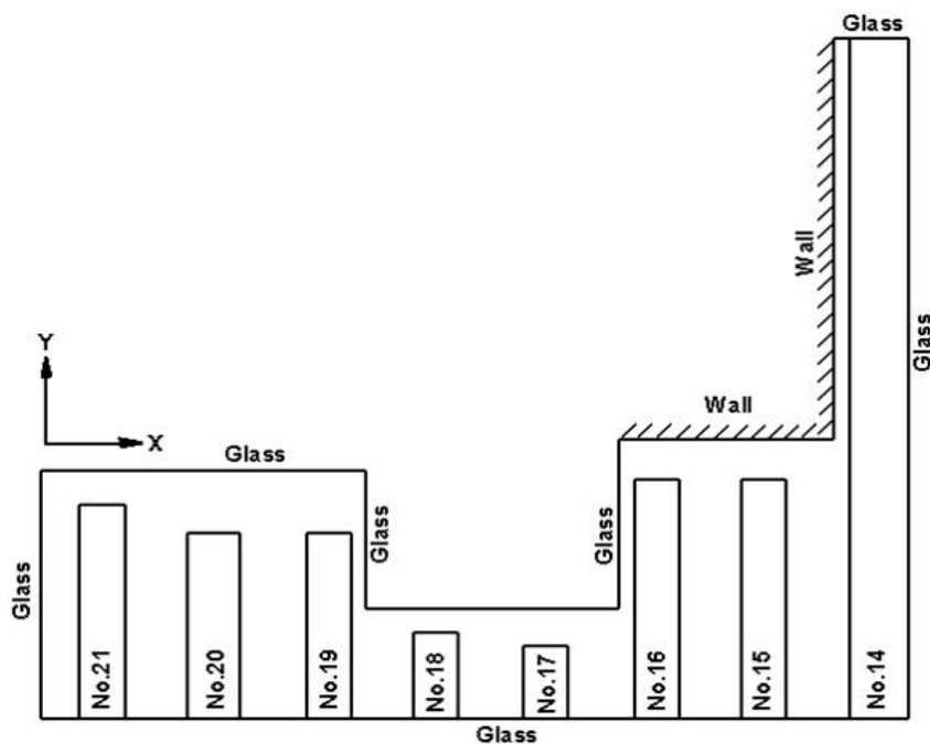
Fig. 1. Draft of model for display hall of Han Yang Mausoleum museum.
