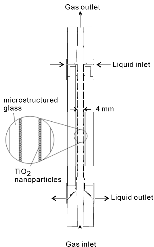
Fig. 1. PPWD: schematic diagram.
